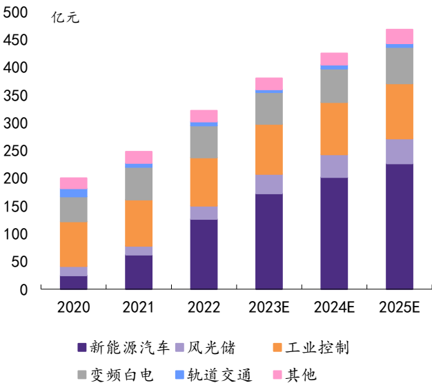
图表：2020-2025年中国IGBT市场结构
