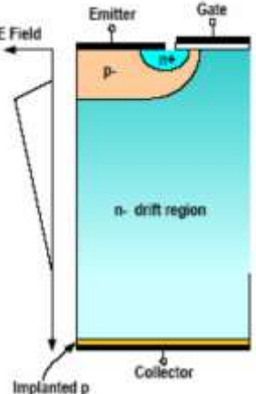
非穿通型（NPT）
