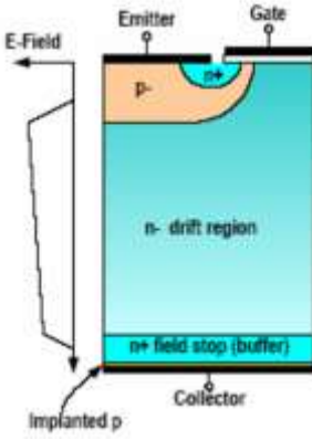
场截止型（FS）
