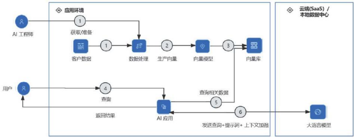
图 8 RAG 流程
