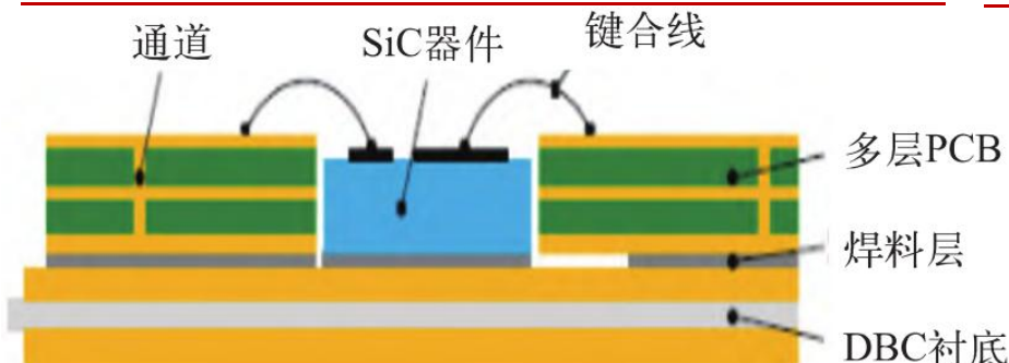
DBC+PCB混合封装结构
