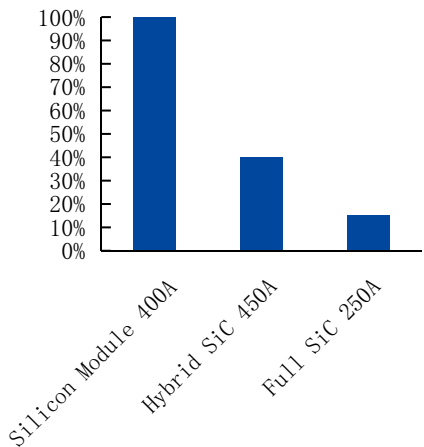
不同功率模块在最大开关频率下的开关损耗
