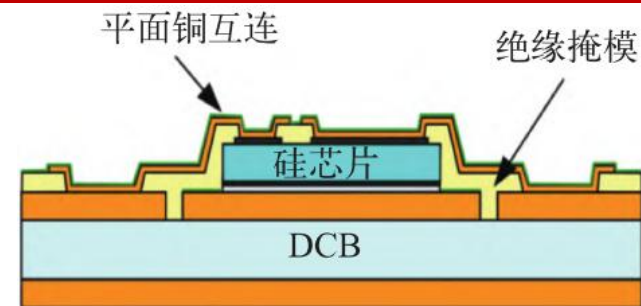
西门子SiPLIT模块横截面
