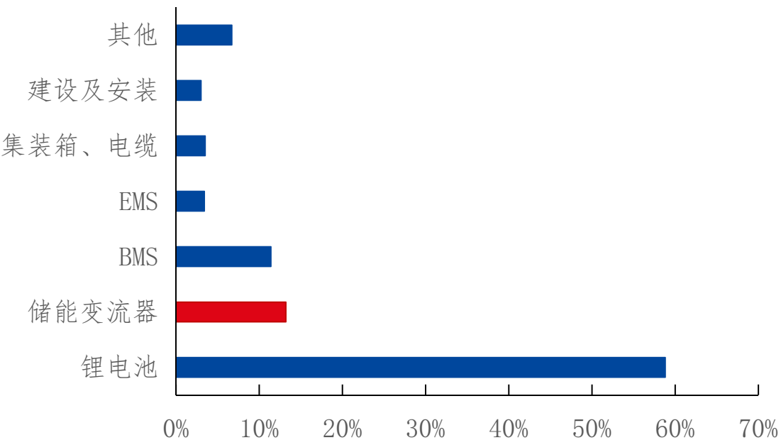
锂电池储能系统成本构成（%）
