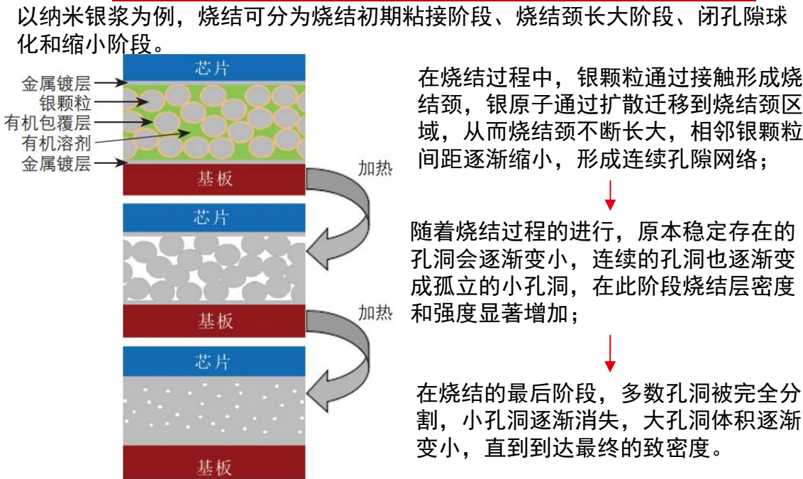
银浆烧结互联示意图
