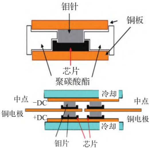
三维（3D）封装结构
