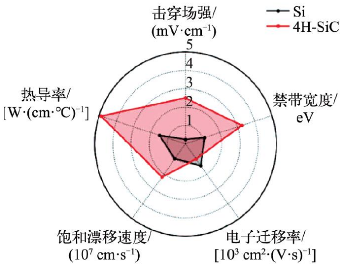
Si和4H-SiC材料的主要特性
