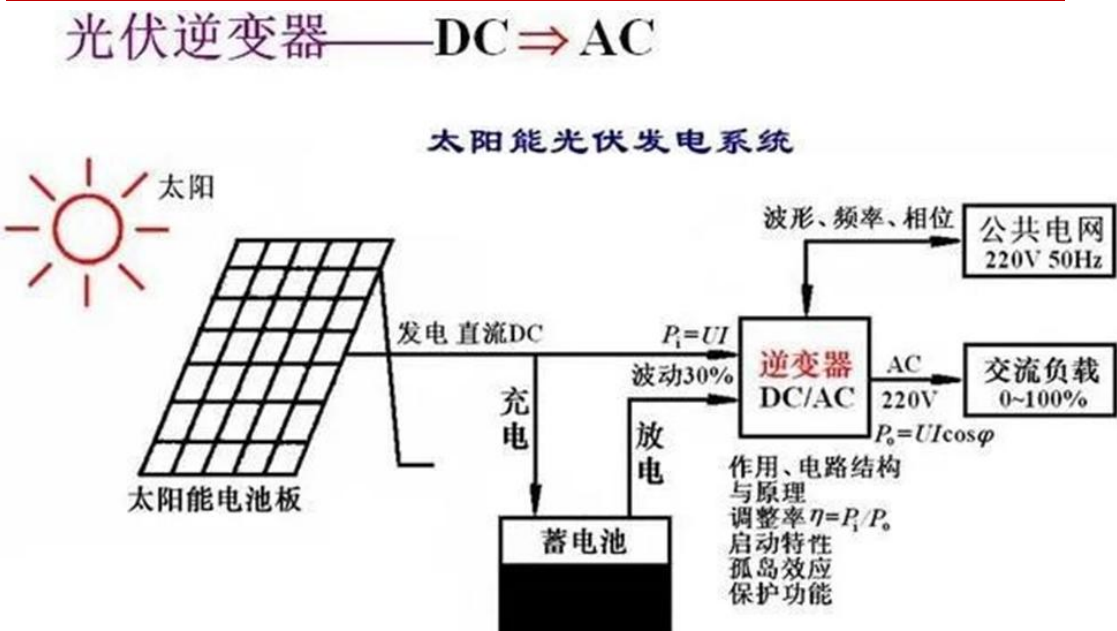
光伏逆变器在太阳能发电系统的作用
