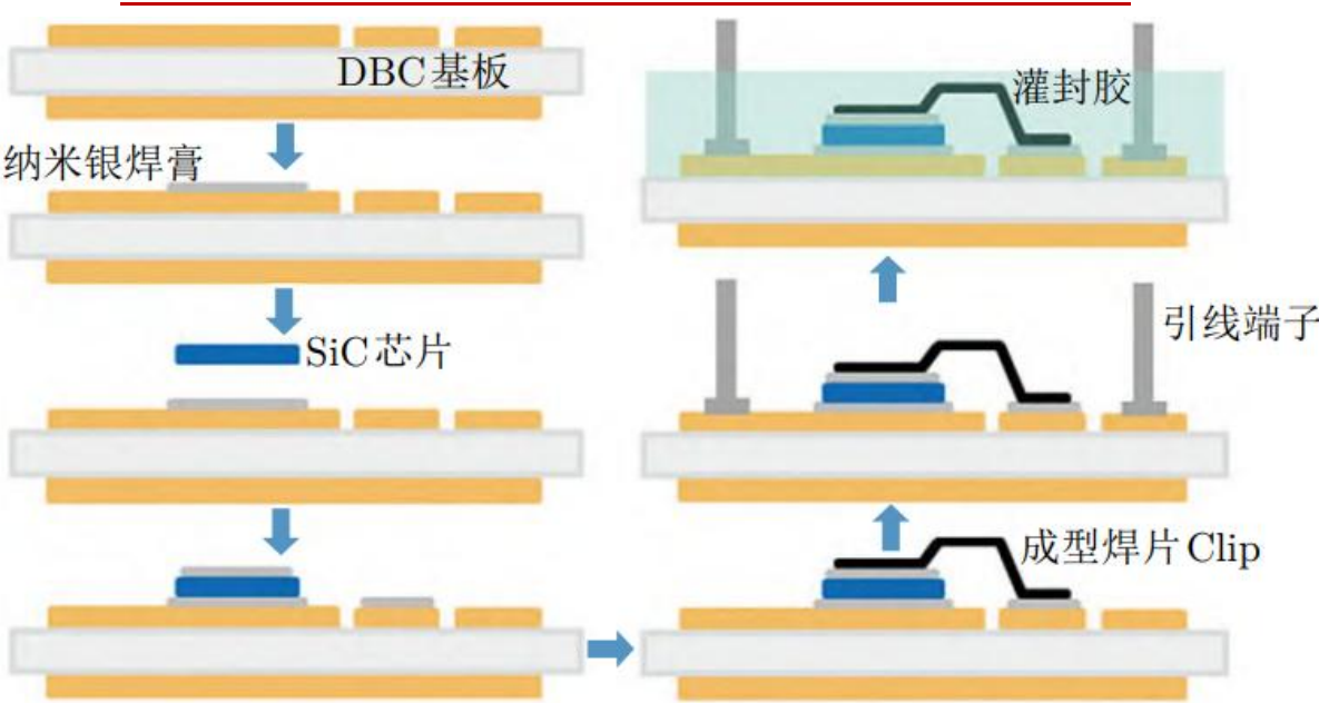
纳米双面银烧结工艺流程
