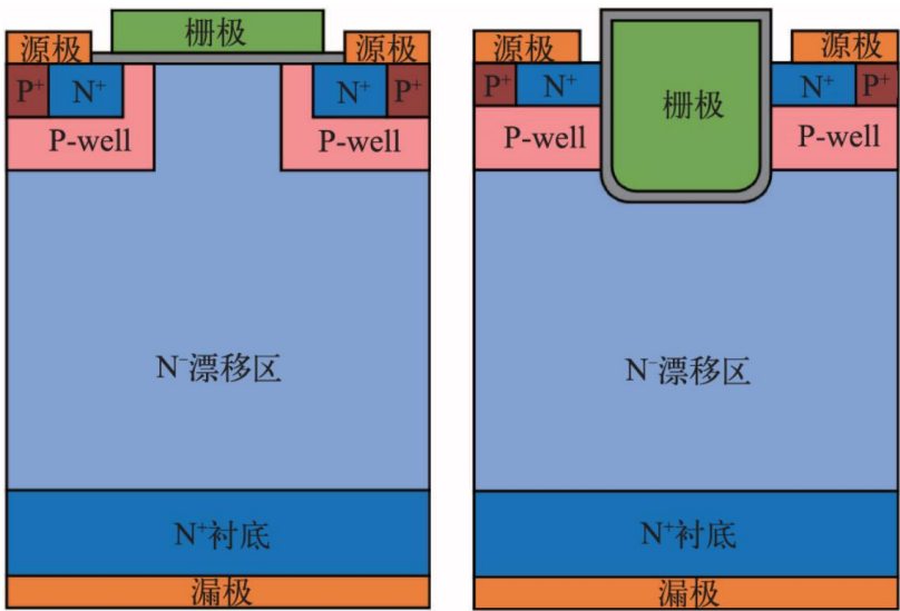
VDMOS（左）和TMOS（右）结构图
